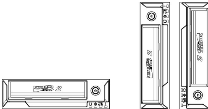
Figura 3: orientaciones de montaje permitidas
