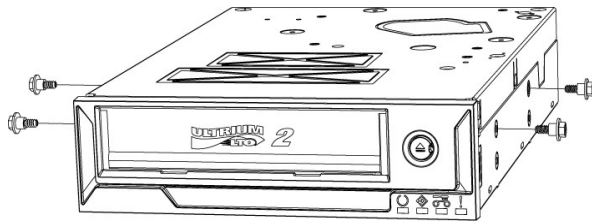
Figura 4: especificaciones de montaje, tornillos con pivote
