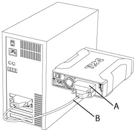
Figura 4: terminación de dispositivos SCSI externos
